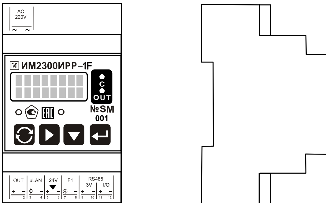
Рисунок 2.8 – Органы управления, индикации и коммутации прибора ИМ2300ИРР-DIN
